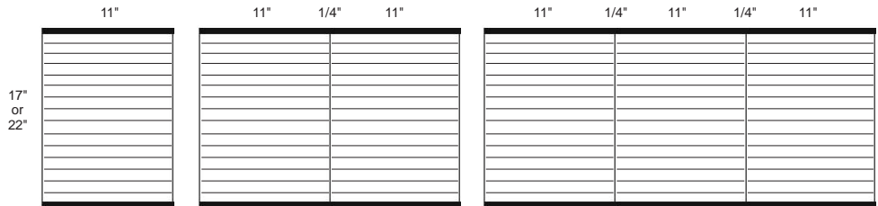
UVR1711-30IS 17"(h) / 14 Bands
